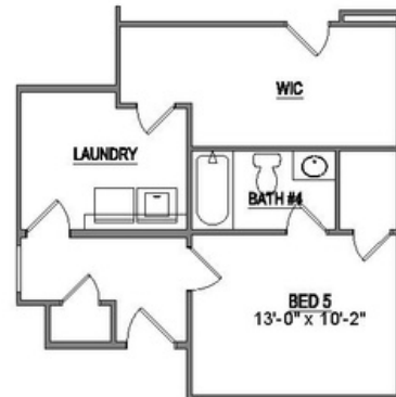
Optional Bed 4 Bath 4
